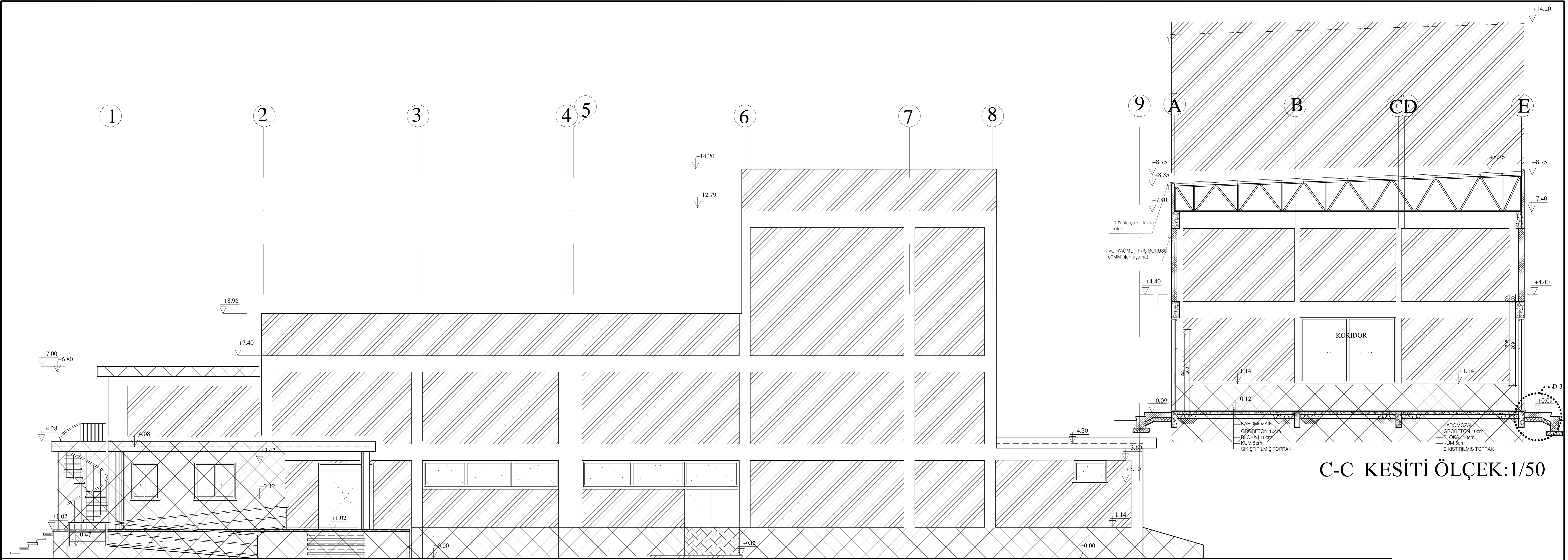
ÖN GÖRÜNÜŞ ÖLÇEK:1/50
