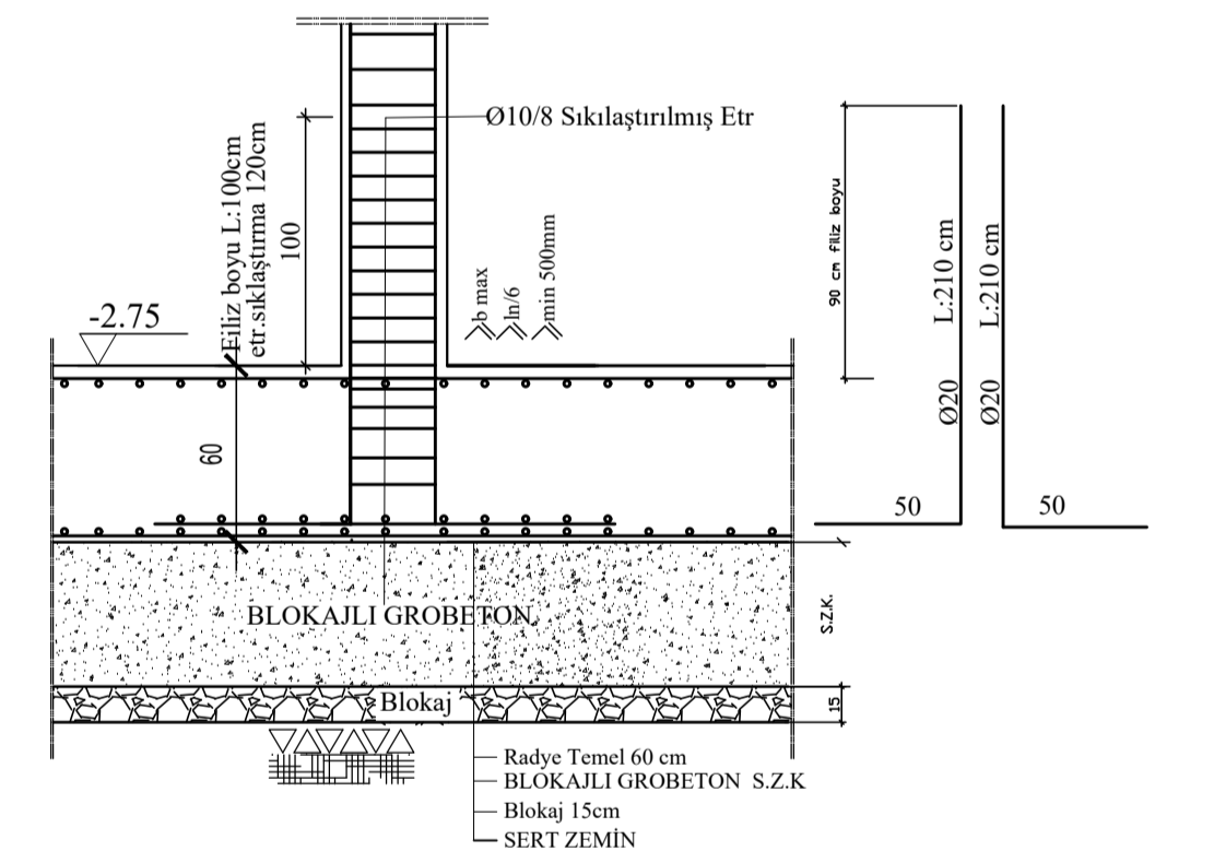
S39 (30/120) RAYLI TEMEL BOY KESİTİ Ö:1/20
