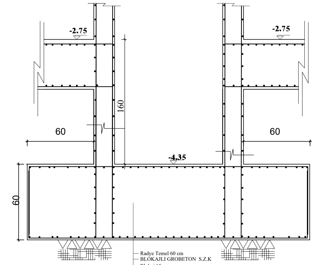
ASANSÖR TEMELİ DETAYI Ö:1/20
